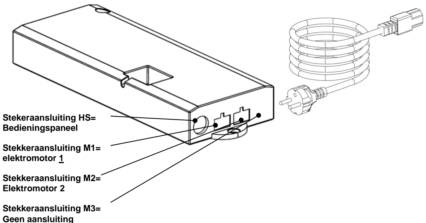
Figuur 2: aansluiting van de stekkers van de elektromotor en het bedieningspaneel in de centrale besturingsunit.
