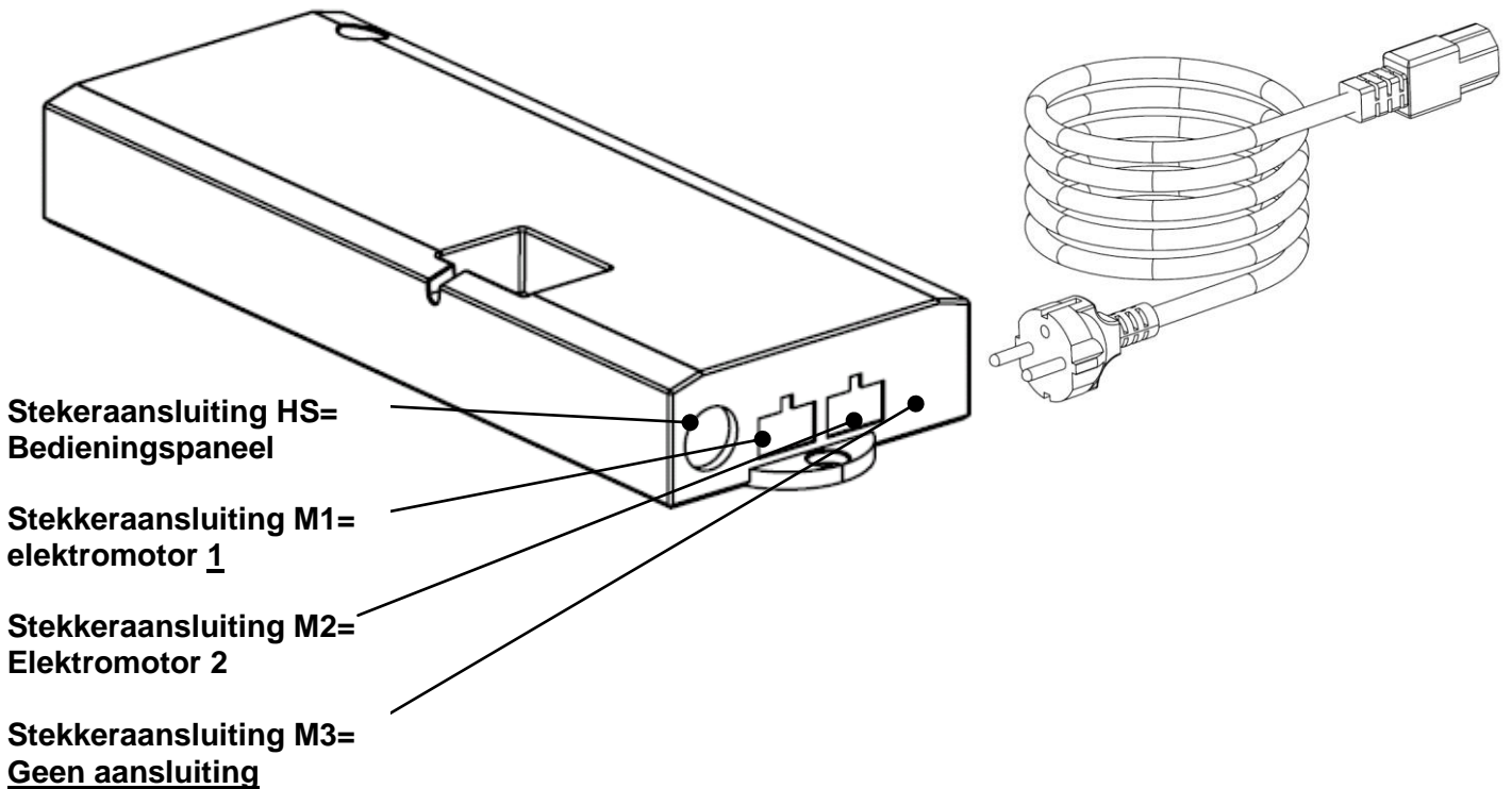
Figuur 3: aansluiting van de stekkers van de elektromotor en het bedieningspaneel in de centrale besturingsunit.
